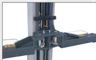
Protezioni in gomma salvaportiera. Arresto rotazione bracci a settori dentati.
