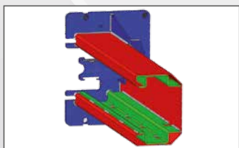
Struttura colonna rinforzata internamente per ridurre la flessione e guida cavi interna.
